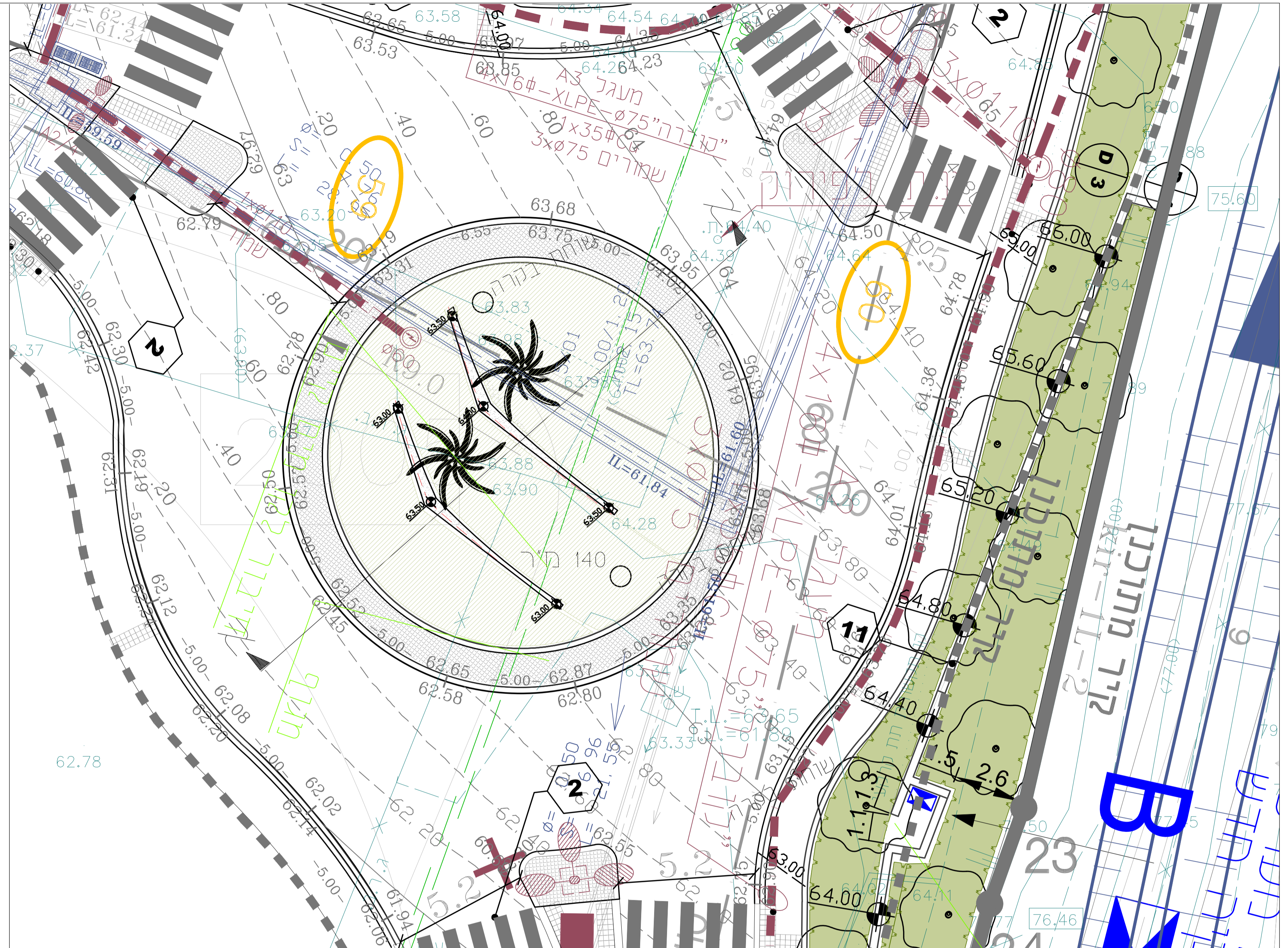
קטע מתכנית 1:100 קני"מ
