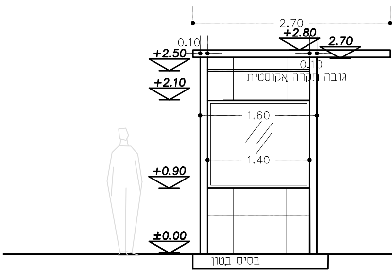
חזית צפונית
