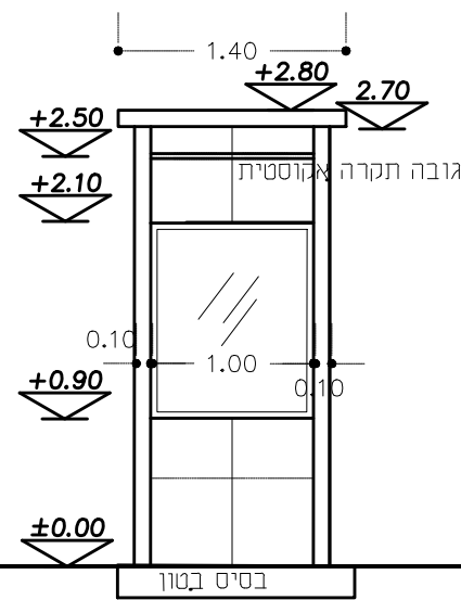
חזית מזרחית
