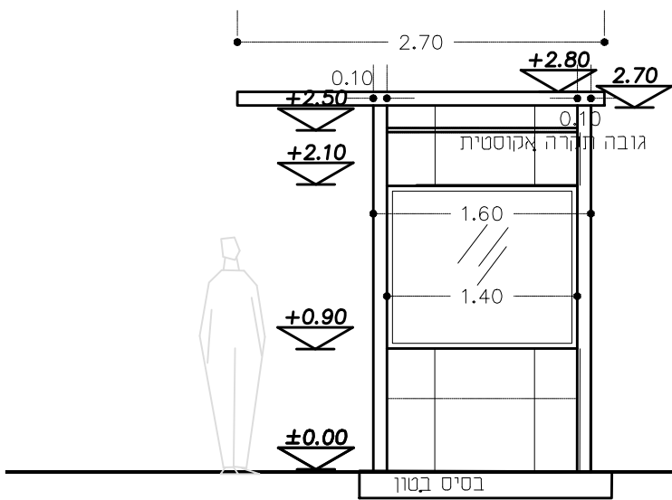
חזית דרומית
