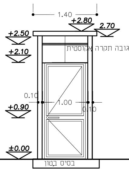
חזית מערבית
